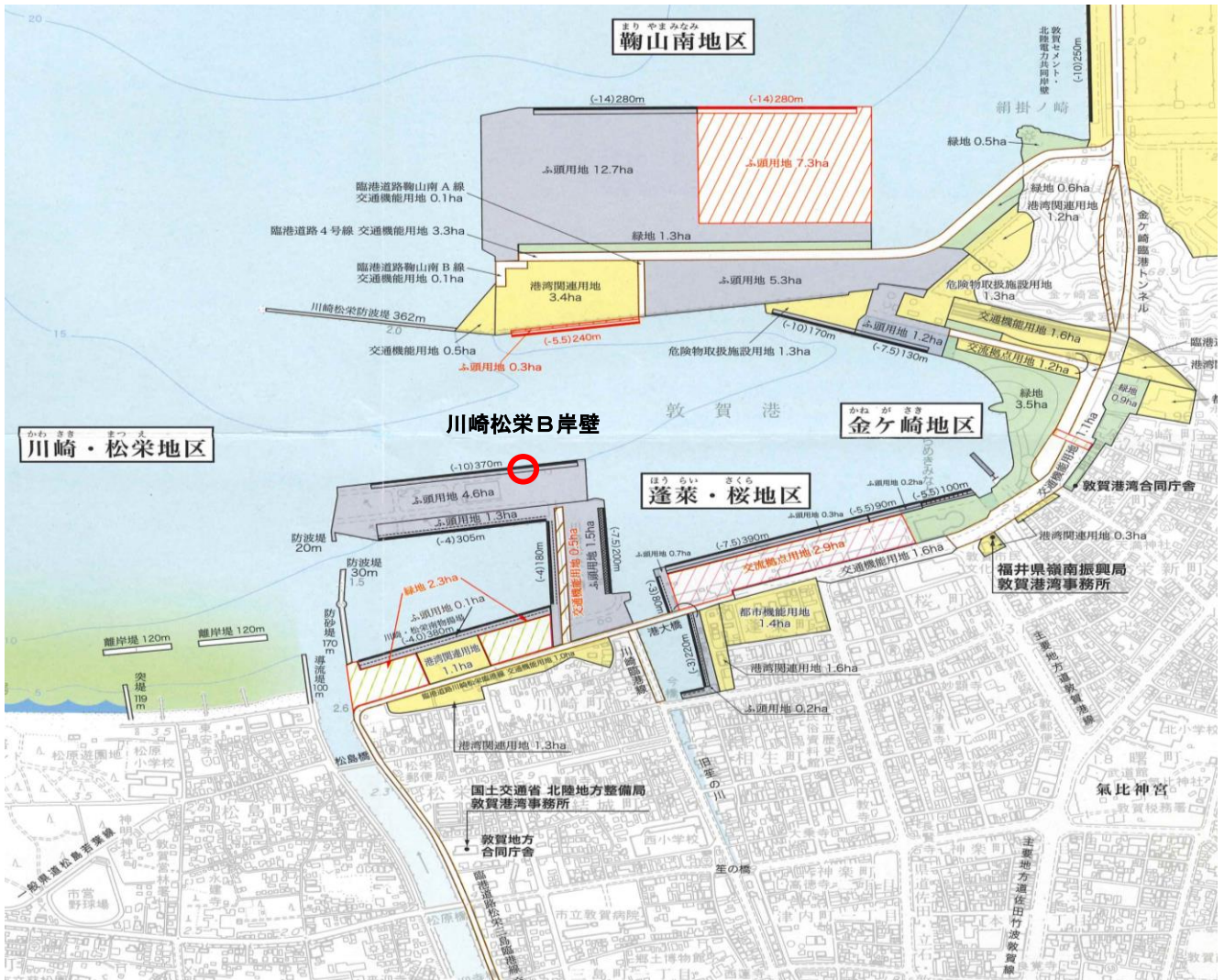
川崎松栄B岸壁 位置図
