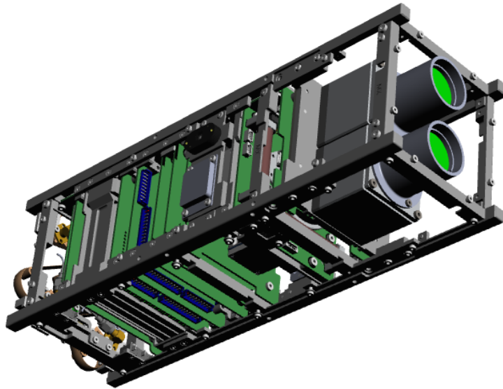
福井県で設計した CAD モデル（春江電子㈱提供）
